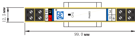
深 114.5mm * 高 22.5mm * 宽 99mm Толщина 114.5мм*ширина 22.5мм*высота 99 мм
